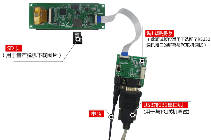
图 1-3 调试工具图
