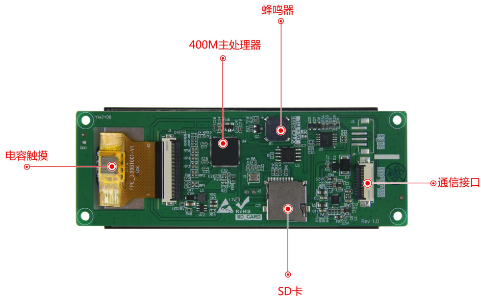
图 1-2 硬件配置图
